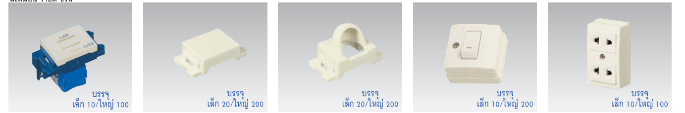
NR3170-8 ตัวรับคอมพิวเตอร์ CAT6 CAT6 Data modular jack WN3020 แผ่นอุดช่องว่าง Blank chip WN3022 แผ่น Telephone wire chip 3 14 มม. Telephone wire chip, 14 mm diameter WSG3001 สวิตช์ล้อย ทางเดียว (สีขาว) Toggle switch "B", single pole 10A 250V~ (White) WKG1092-250 ตัวรับคู่ เสียบขากลมแบน (สีขาว) Universal duplex receptacle
