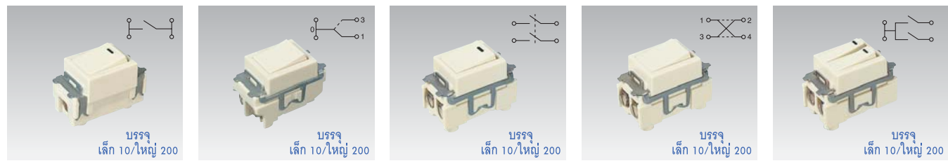
WNG5001-701 สวิตช์ทางเดียว Switch "B", single pole 16AX250V~ WNG5002-701 สวิตช์ 3 ทาง Switch "C", 3-way 16AX250V~ WNG5003-7 สวิตช์ตัด 2 ขั้วสาย Switch "D", double pole 10A 250V~ WNG5004-7 สวิตช์ 4 ทาง Switch "E", 4-way 10A 250V~ WNG5021-7 สวิตช์คู่ ทางเดียว Twin switch "B", single pole 10A 250V~
