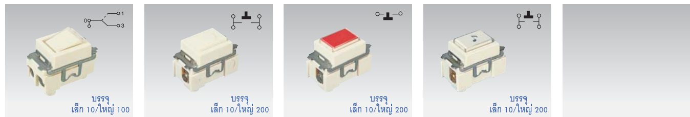
WNG5062-701 สวิตช์ 3 ทาง พร้อมฝาครอบใส Appellation switch "C", 3-way 16AX250V~ WNG5401-7K สวิตช์กด (1 NO) Pushbutton "B", single pole 10A 250V~ WNG5460-7K สวิตช์กดปิด (1 NC) พร้อมฝาครอบใส Appellation pushbutton NC contact type 10A 250V~ WNG5461-7 สวิตช์กดเปิด (1 NO) พร้อมฝาครอบใส Appellation pushbutton "B", single pole 10A 250V~
